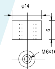
КЛЕММ Т16
