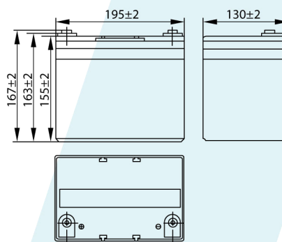
КЛЕММ Т16
